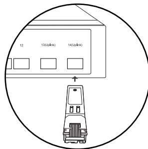
电口模块插入交换机的SFP插槽
